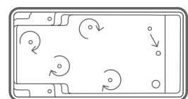
Cyrkulacja wody przy użyciu dysz VANTAGE
